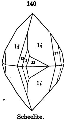
Scheelite.
